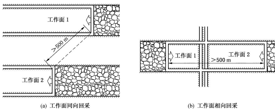
图9 冲击地压危险煤层采掘工作面距离要求
